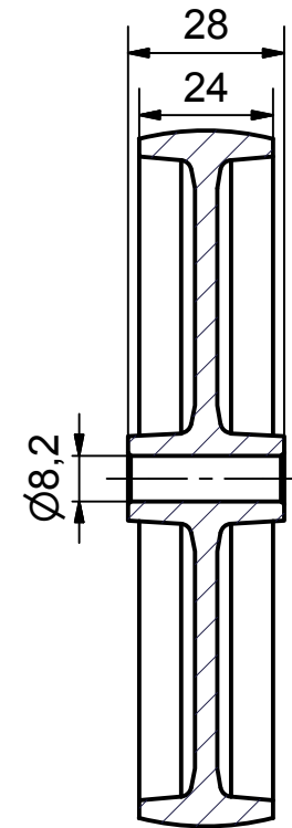
SECTION A-A'
